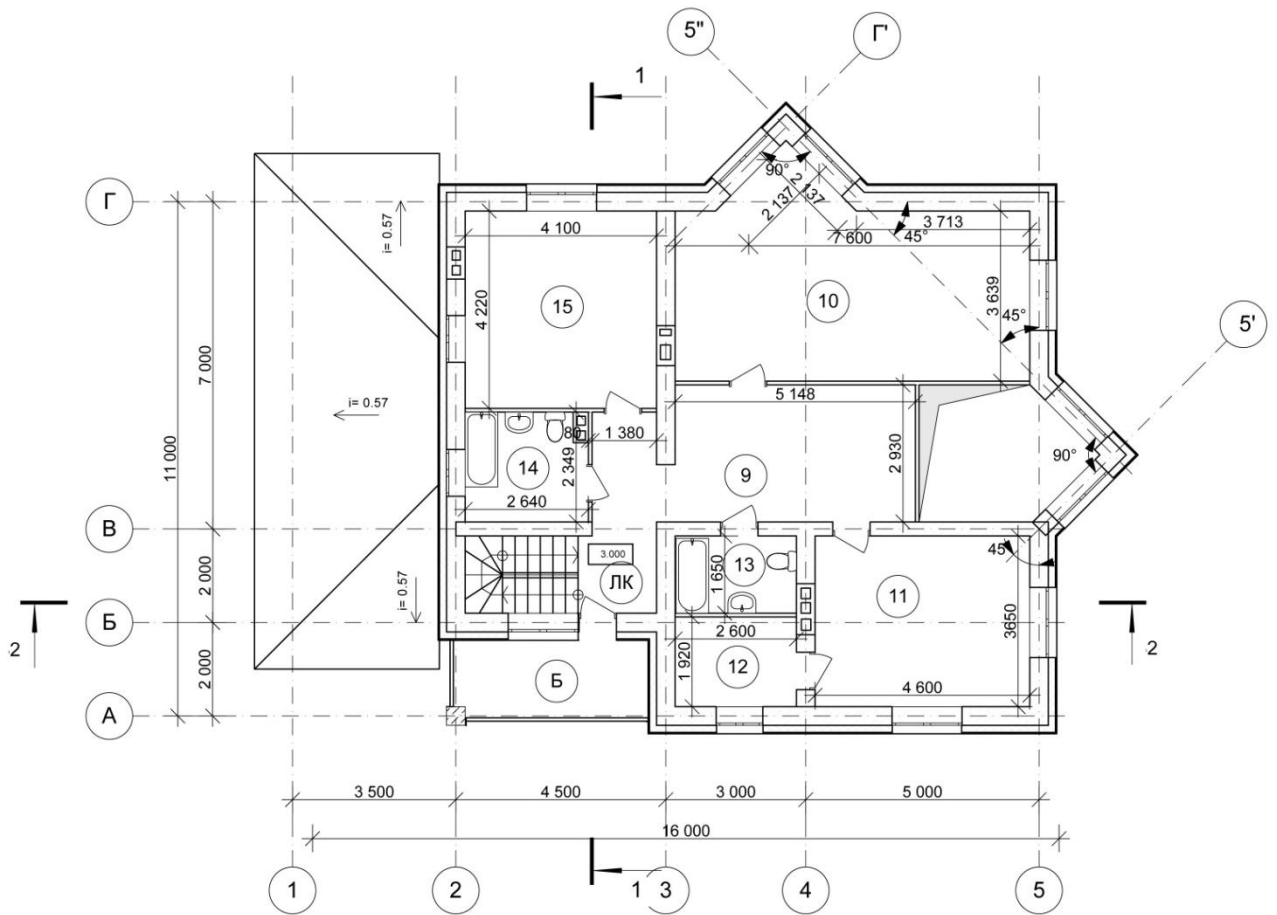
Экспликация 2 этажа
